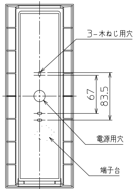
取付部
