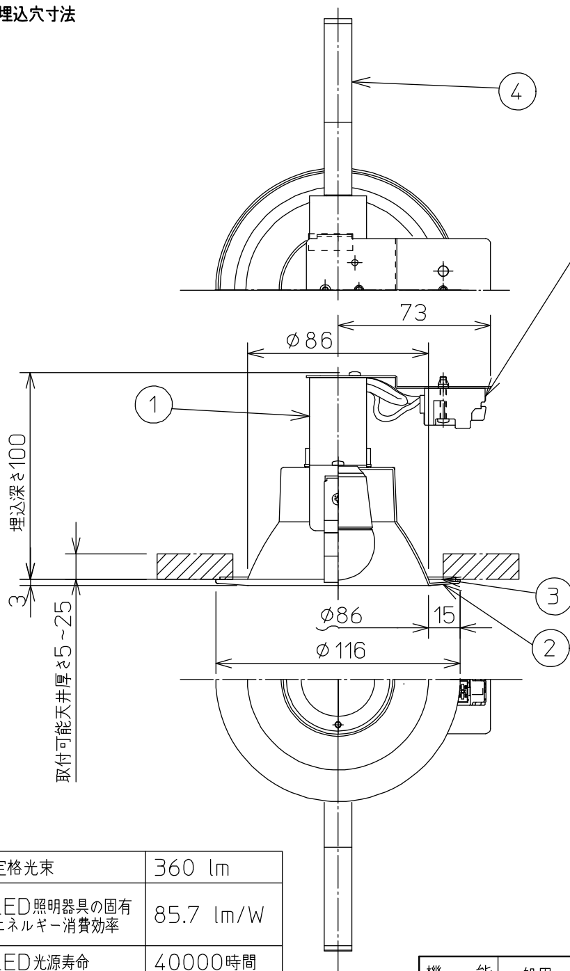
埋込穴寸法
