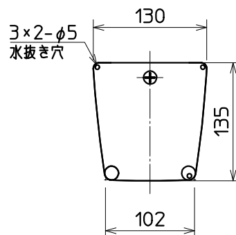
断面詳細図
