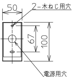
取付部
