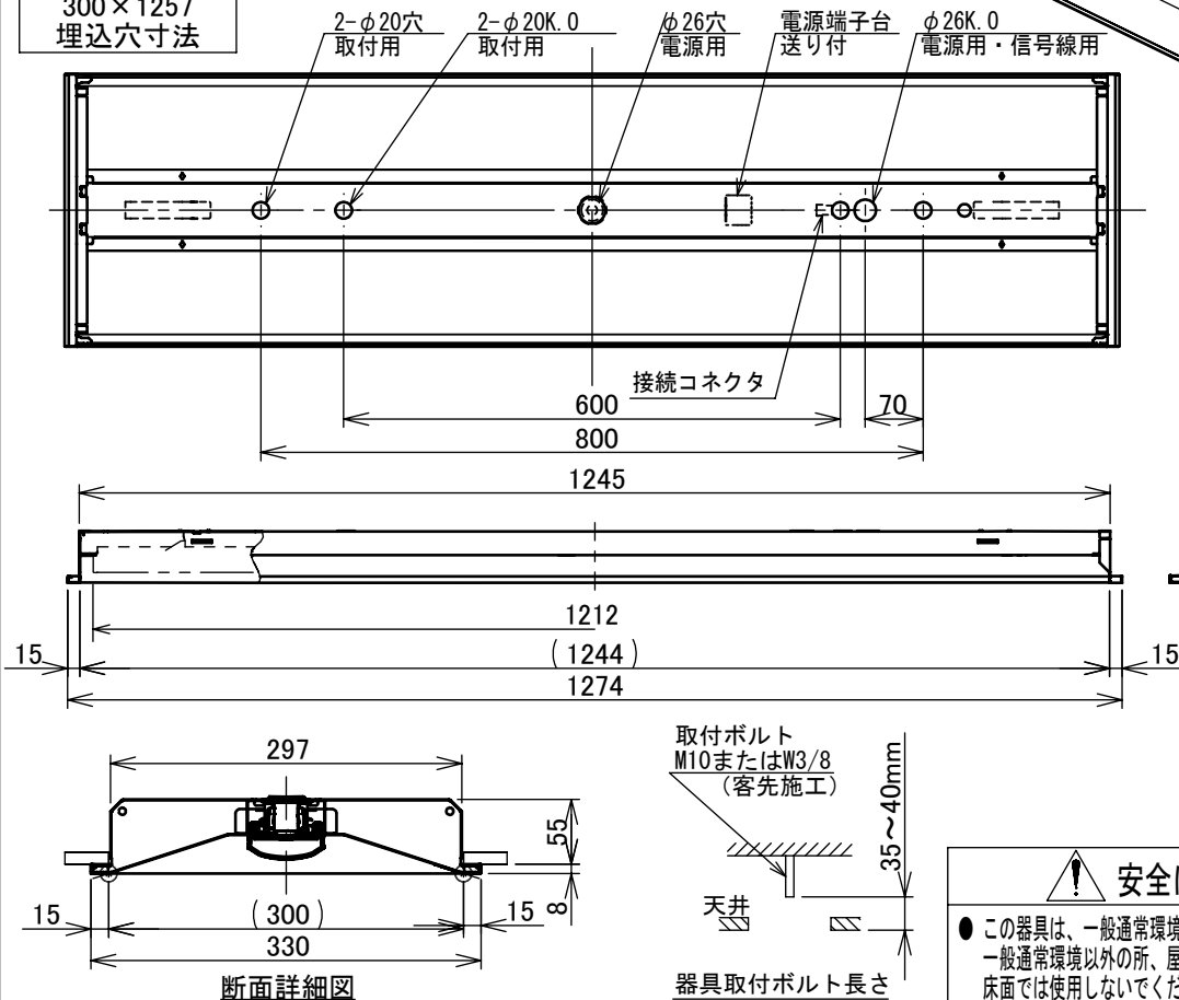
断面詳細図
