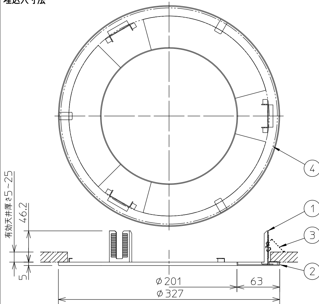
埋込穴寸法
