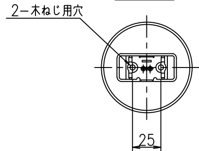
取付部詳細
