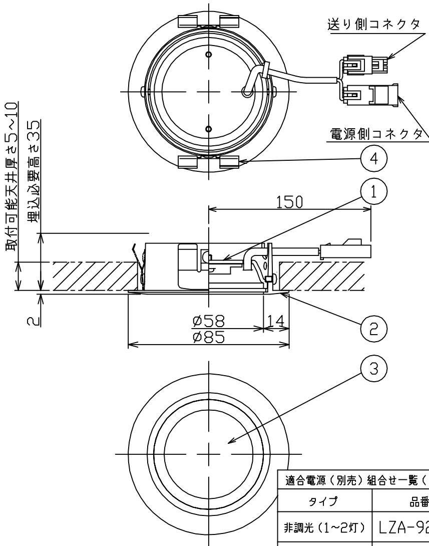
埋込穴寸法
