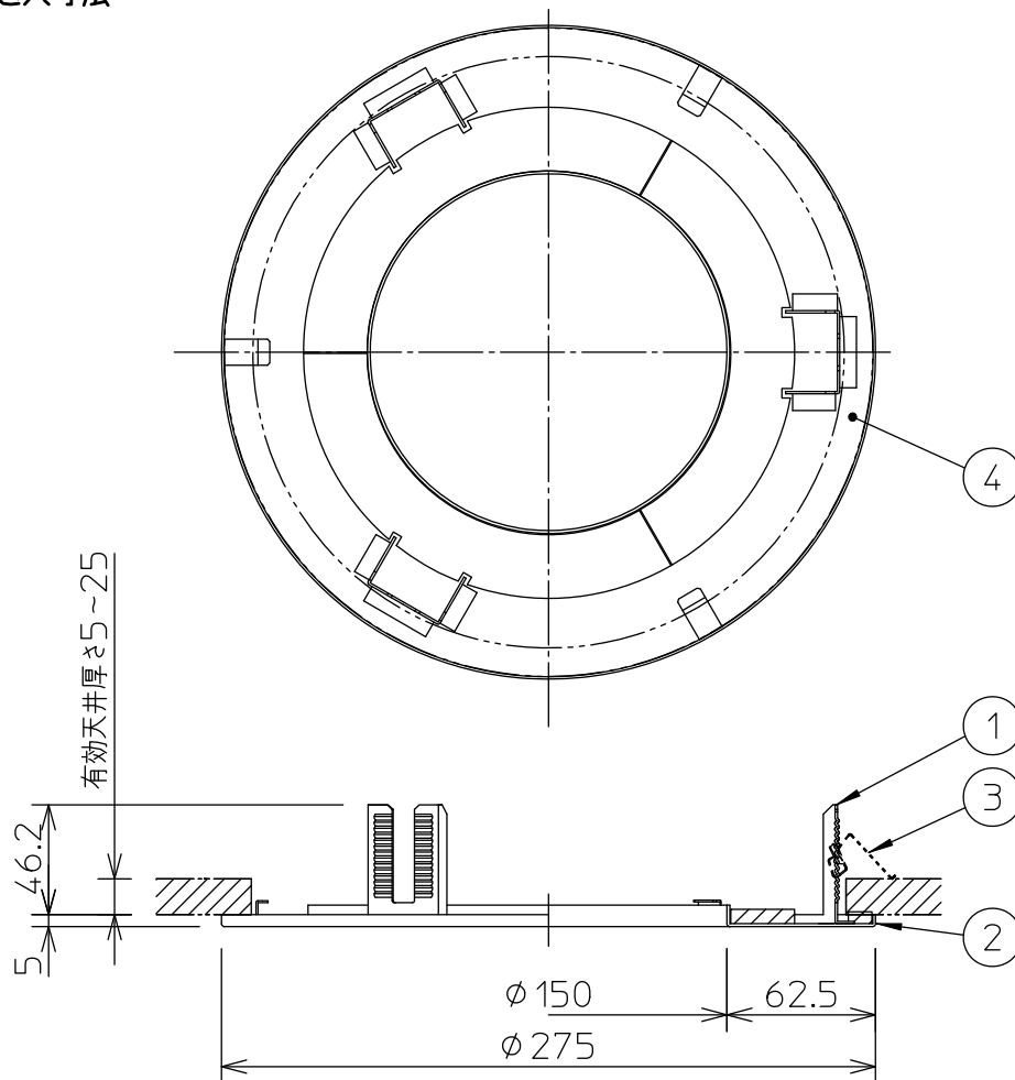
埋込穴寸法
