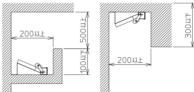
最小施工寸法
