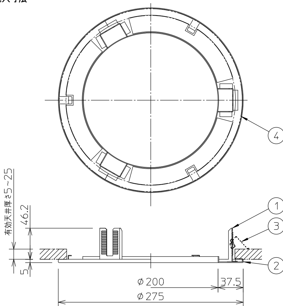
埋込穴寸法
