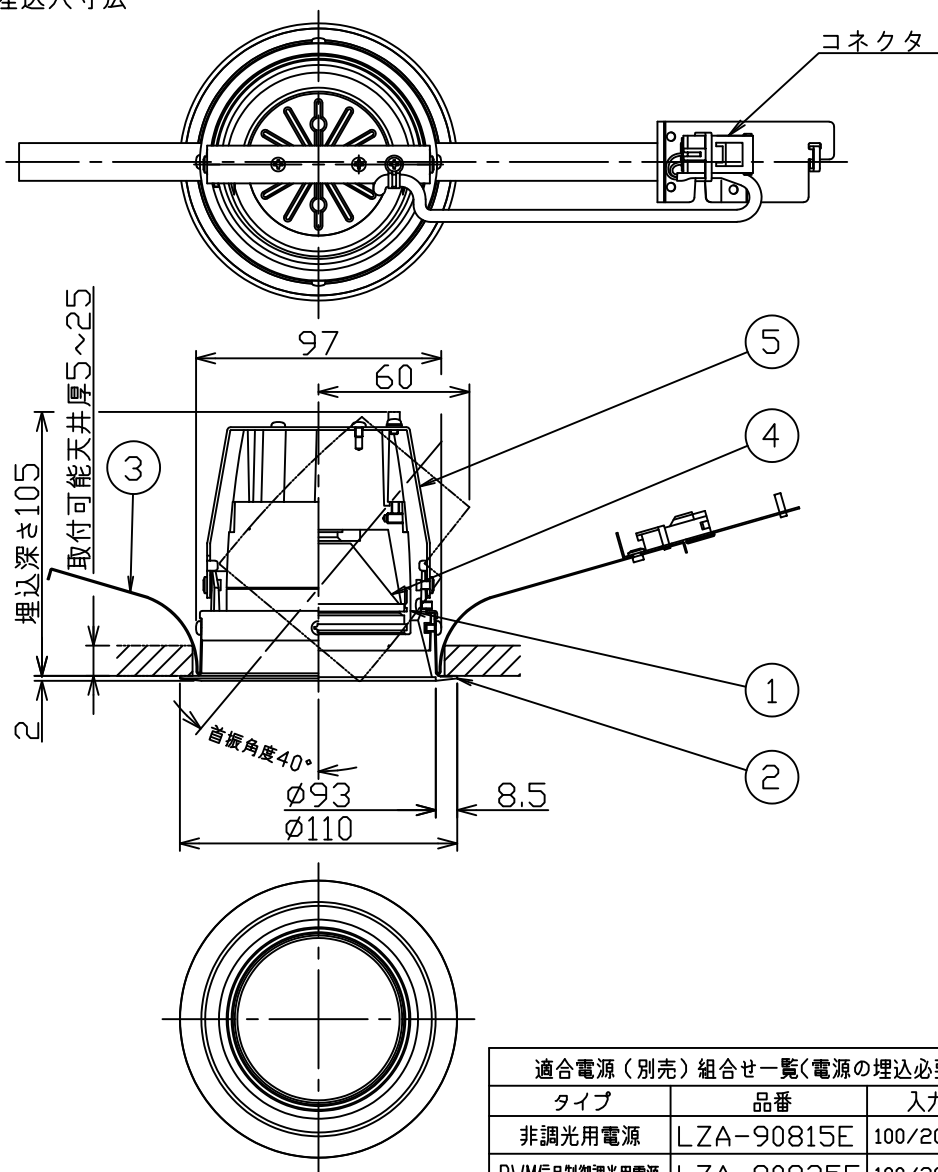
埋込穴寸法
