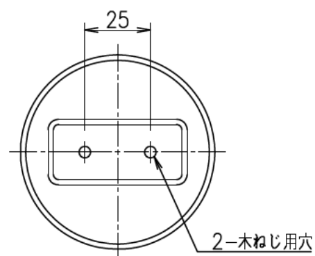
取付部詳細図
