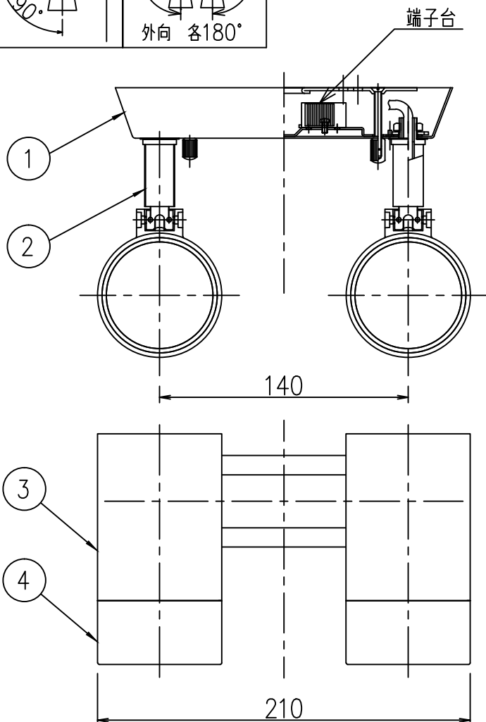
取付部
