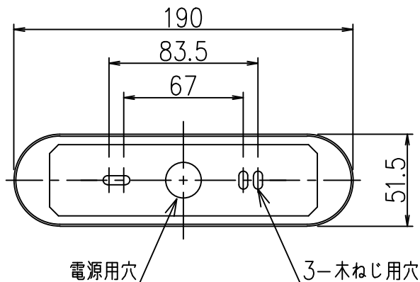
取付部
