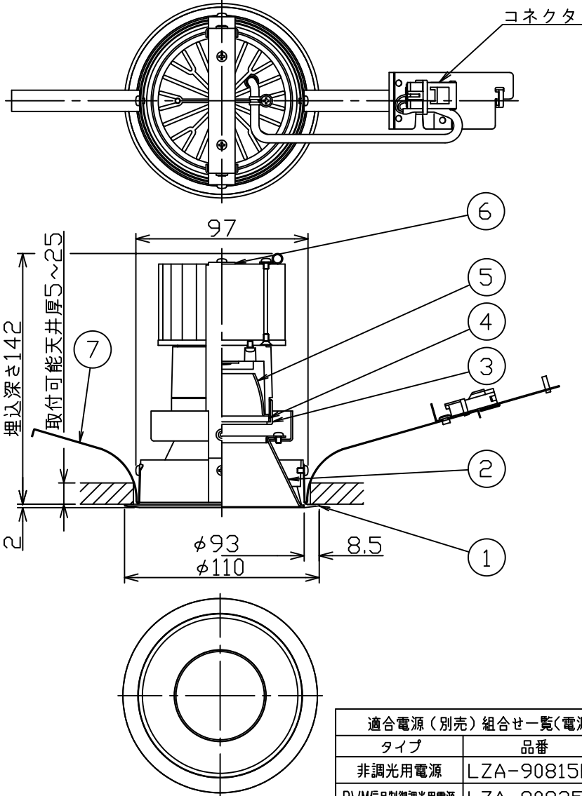
埋込穴寸法
