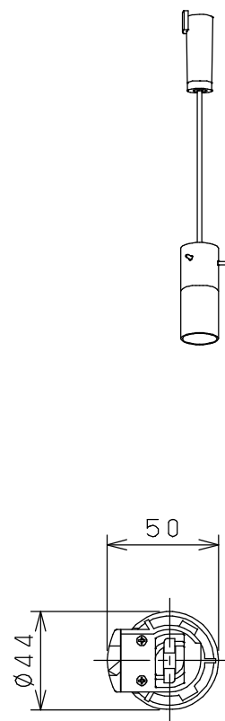
取付部詳細
