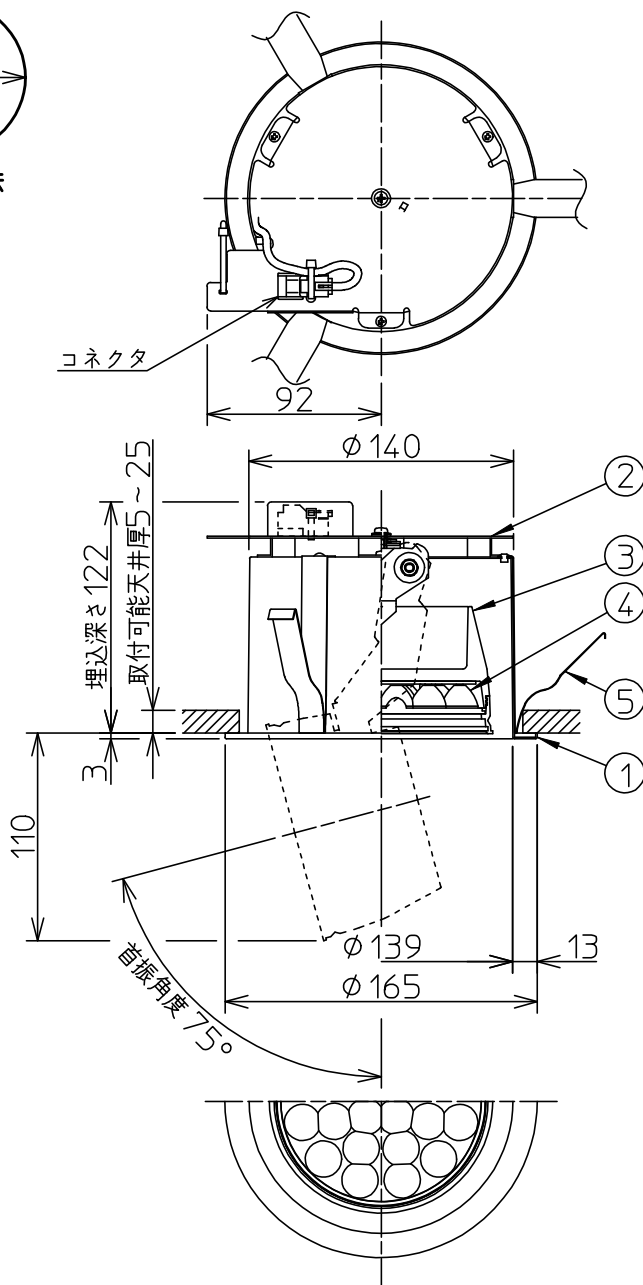
埋込穴寸法
