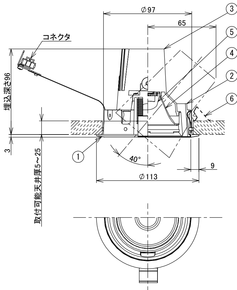
埋込穴寸法
