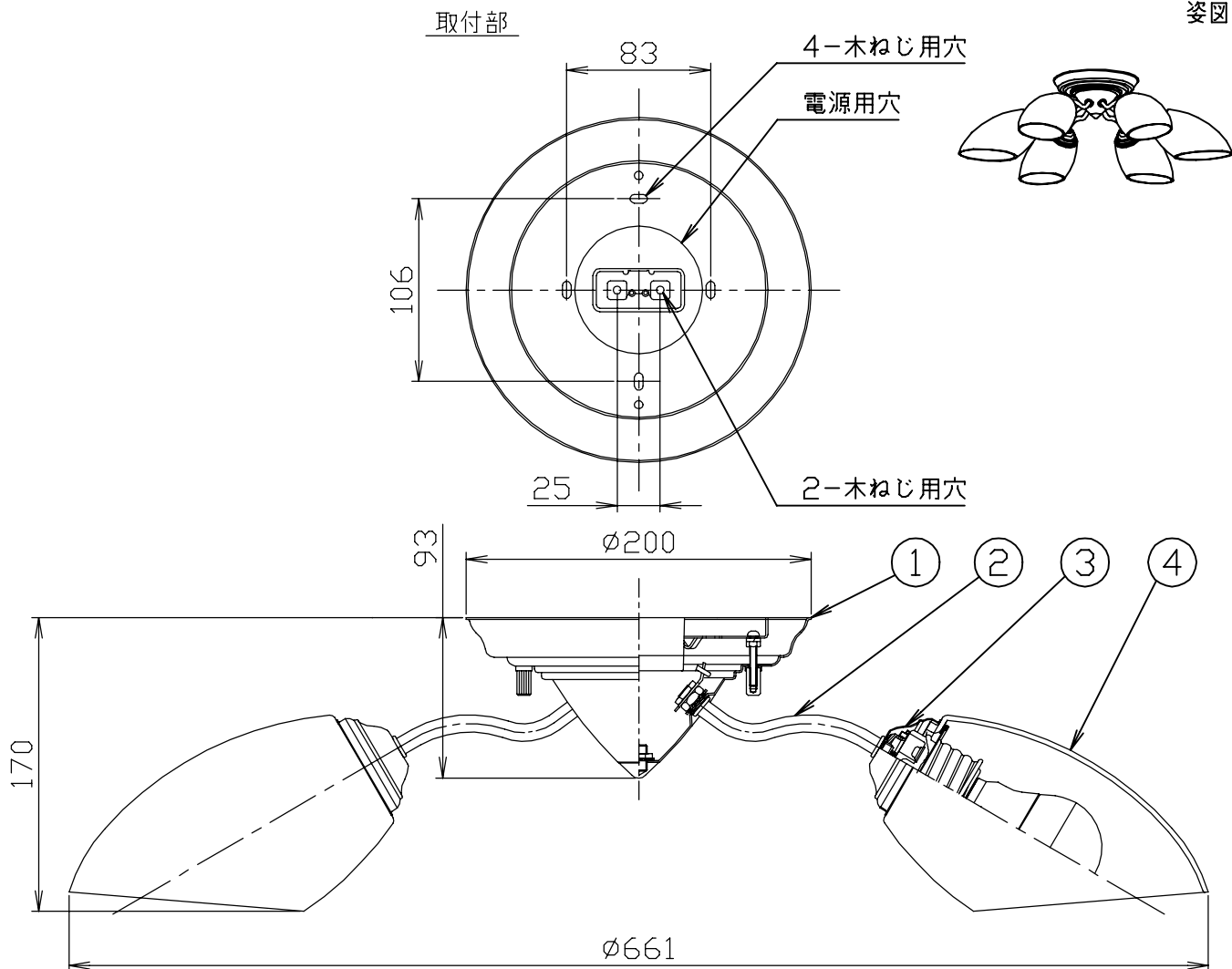
灯具配置図
