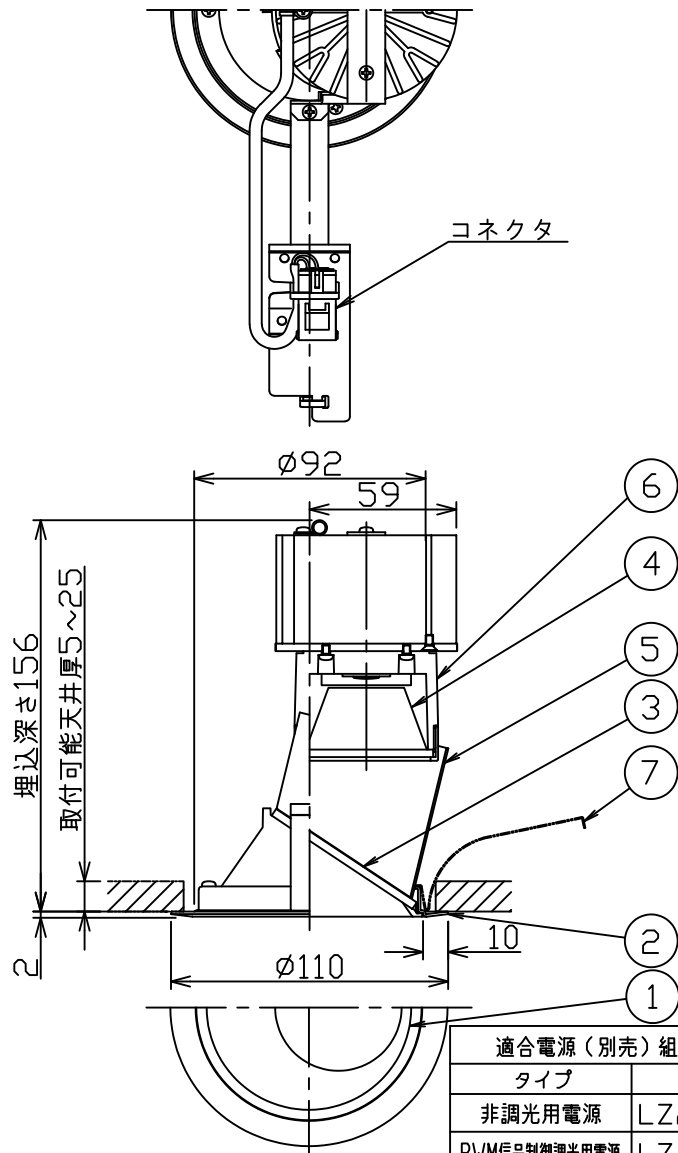
埋込穴寸法
