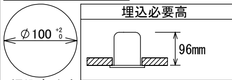
埋込穴寸法
