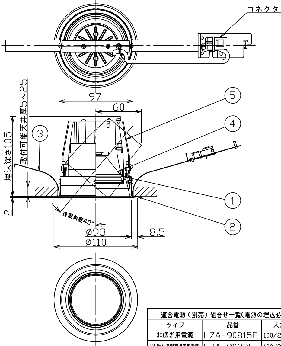
埋込穴寸法
