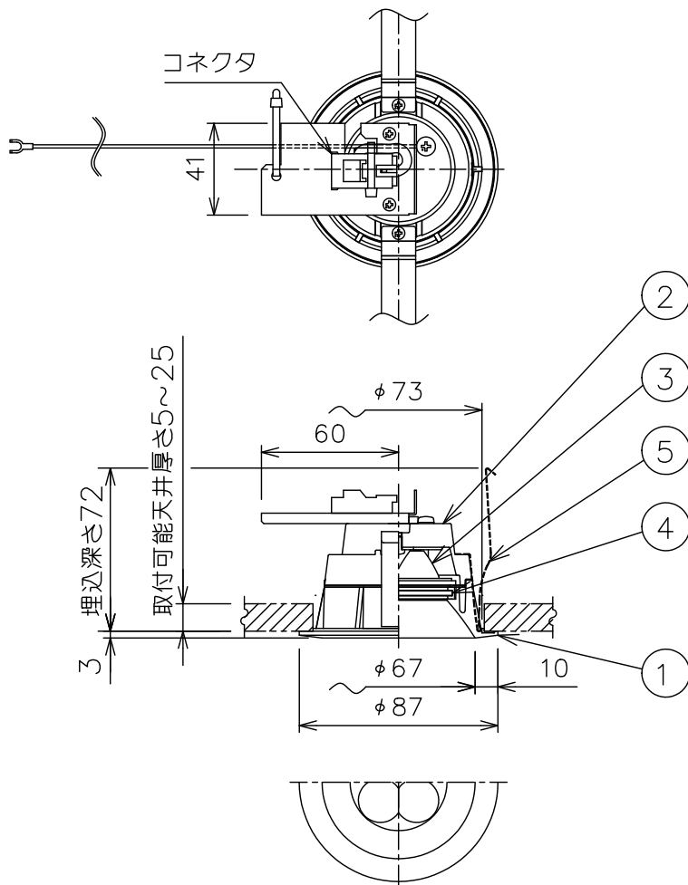
埋込穴寸法
