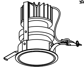
姿図
