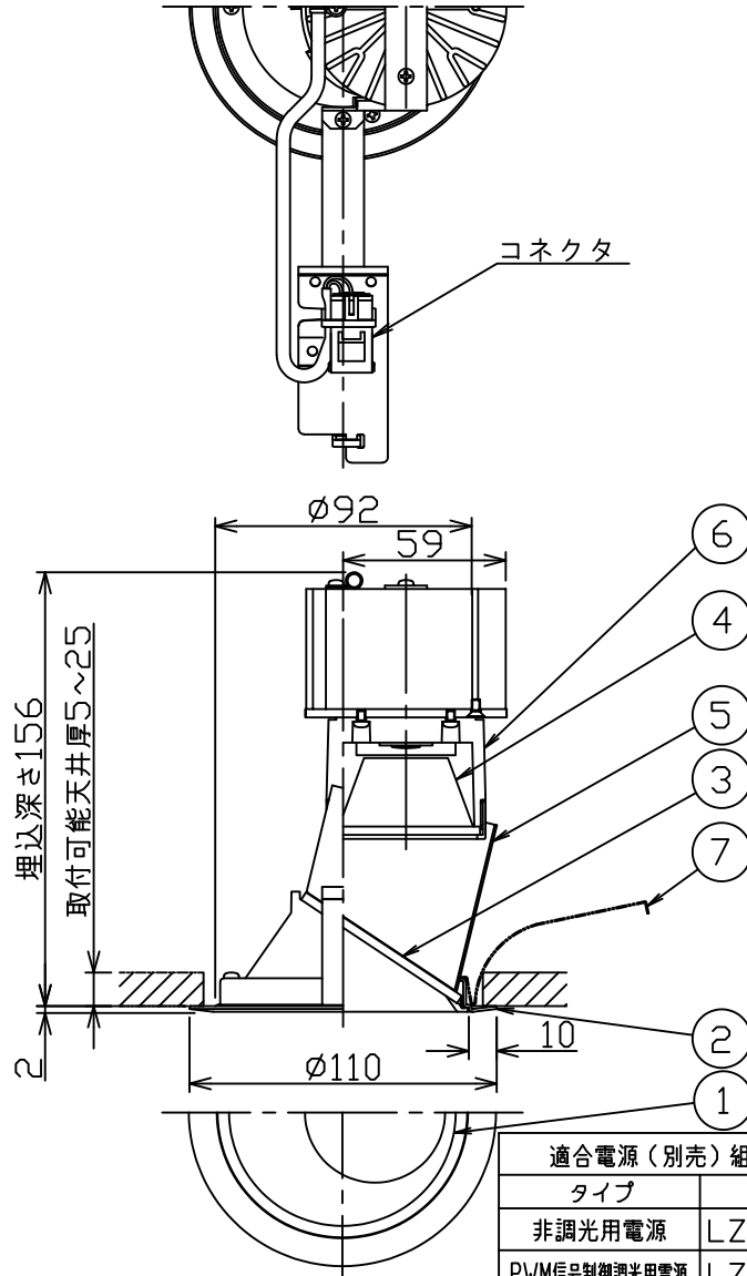
埋込穴寸法
