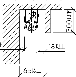
天井取付時(上下可動)
