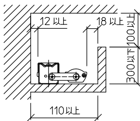
床面取付時(左右可動)
