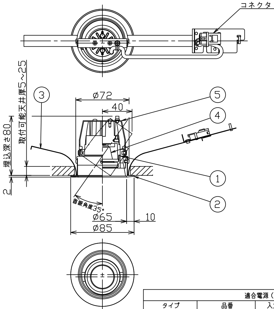
埋込穴寸法
