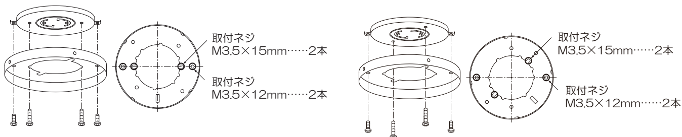
引掛埋込ローゼット
