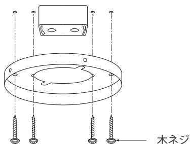
角形引掛シーリング
