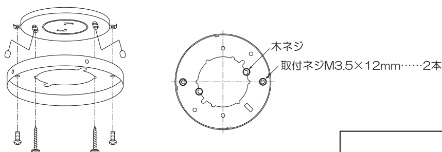
引掛露出ローゼット
