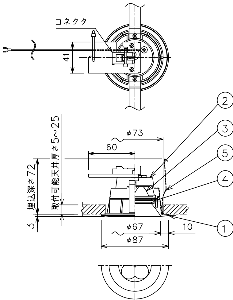
埋认穴寸法
