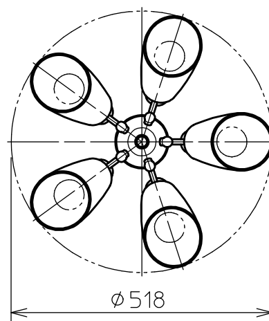
灯具配置図
