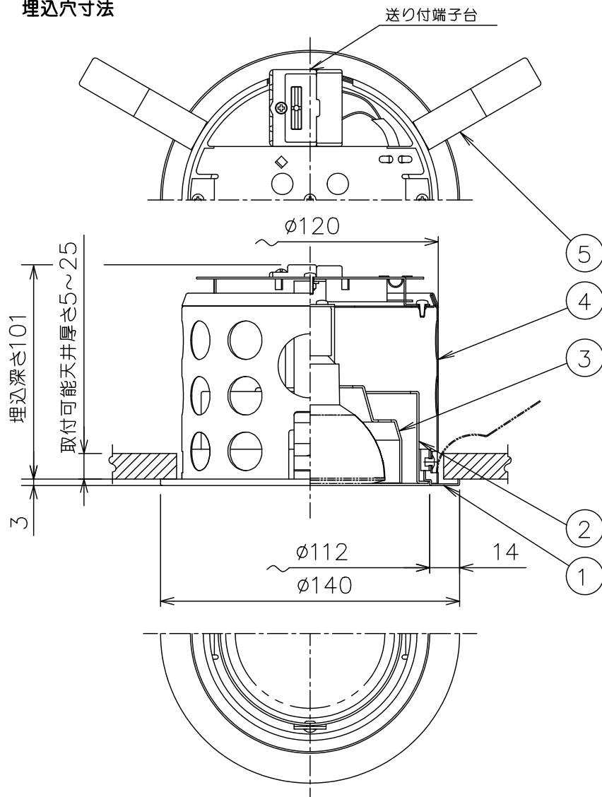
埋込穴寸法
