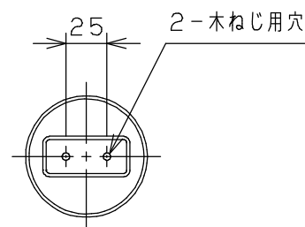
取付部詳細
