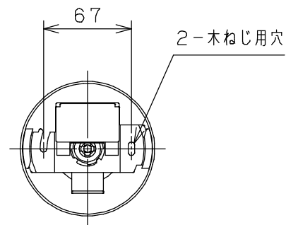
取付部詳細
