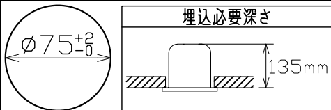
埋込穴寸法
