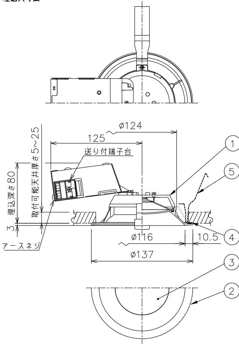
埋込穴寸法
