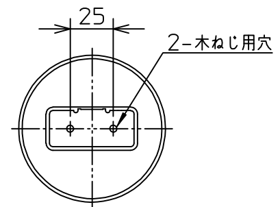
取付部詳細
