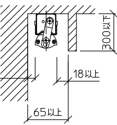
天井取付時(上下可動)
