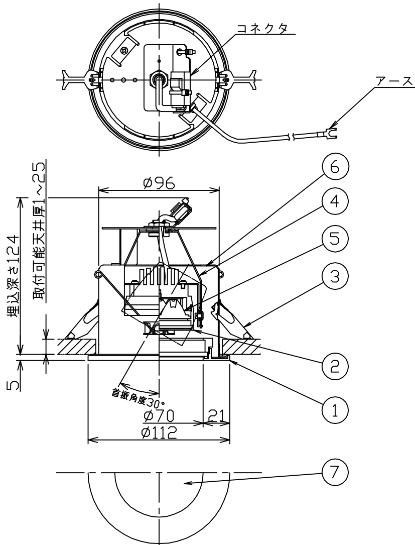
埋込穴寸法
