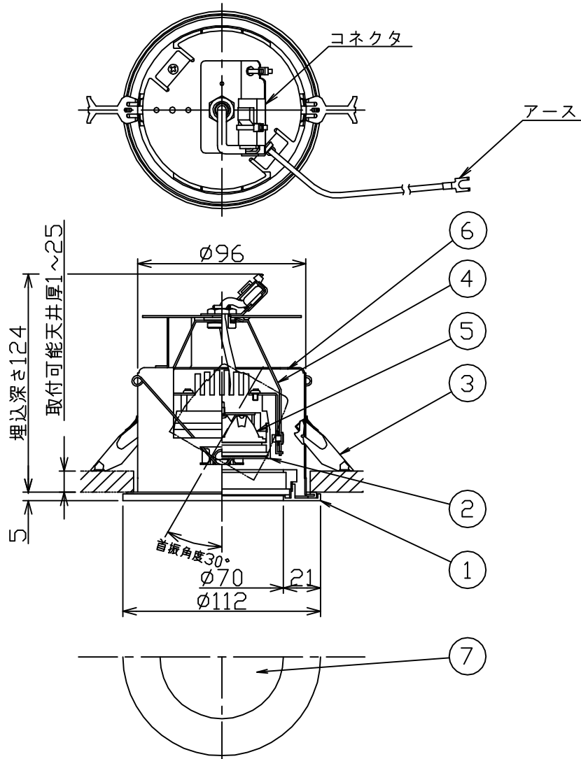
埋込穴寸法
