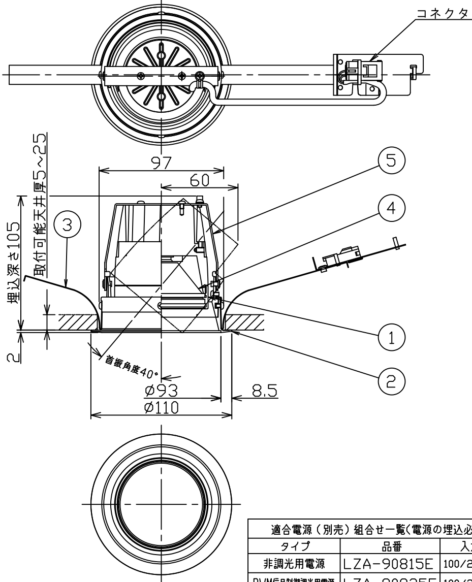
埋込穴寸法
