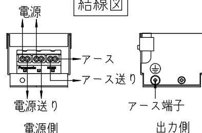
結線図
