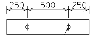
2-木ねじ用穴 取付部詳細
