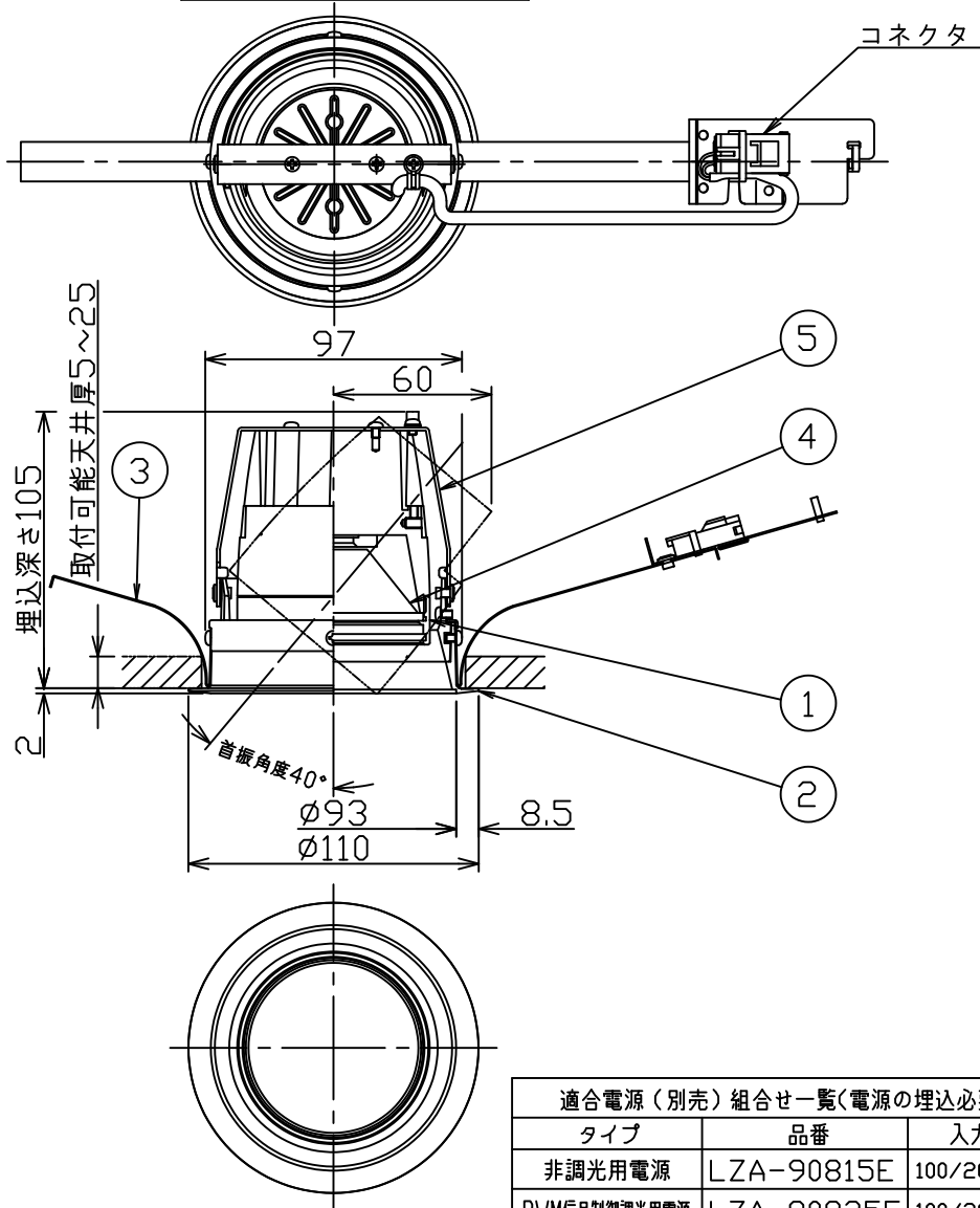
埋込穴寸法
