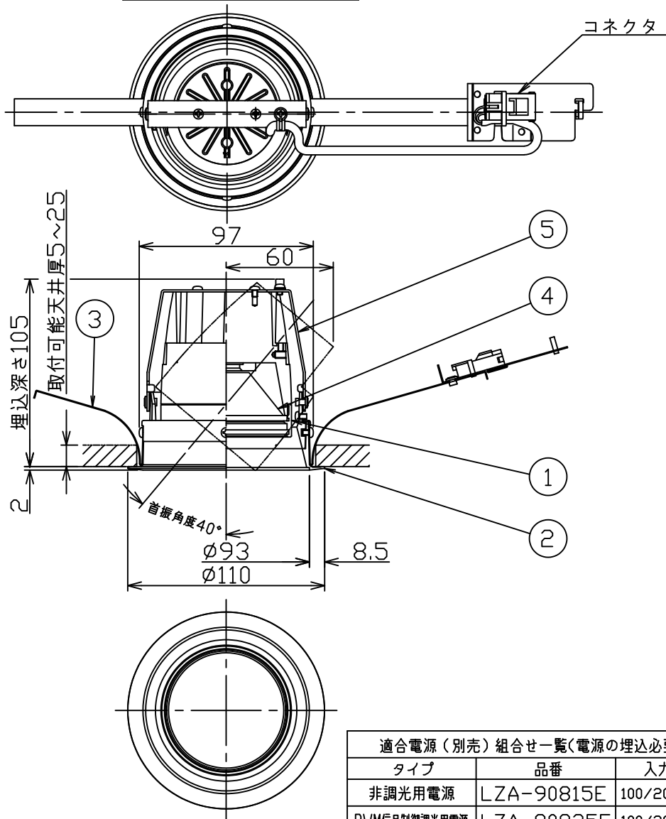
埋込穴寸法
