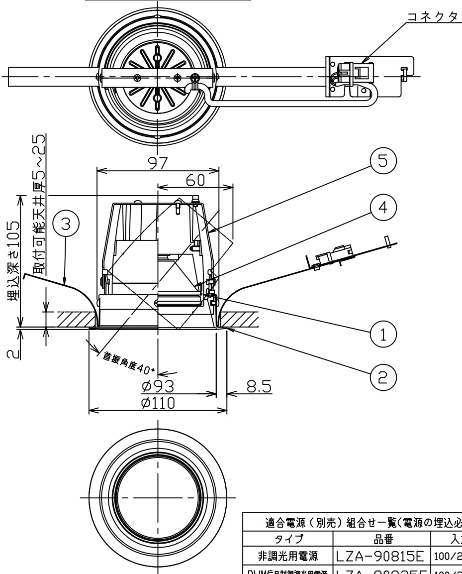
埋込穴寸法
