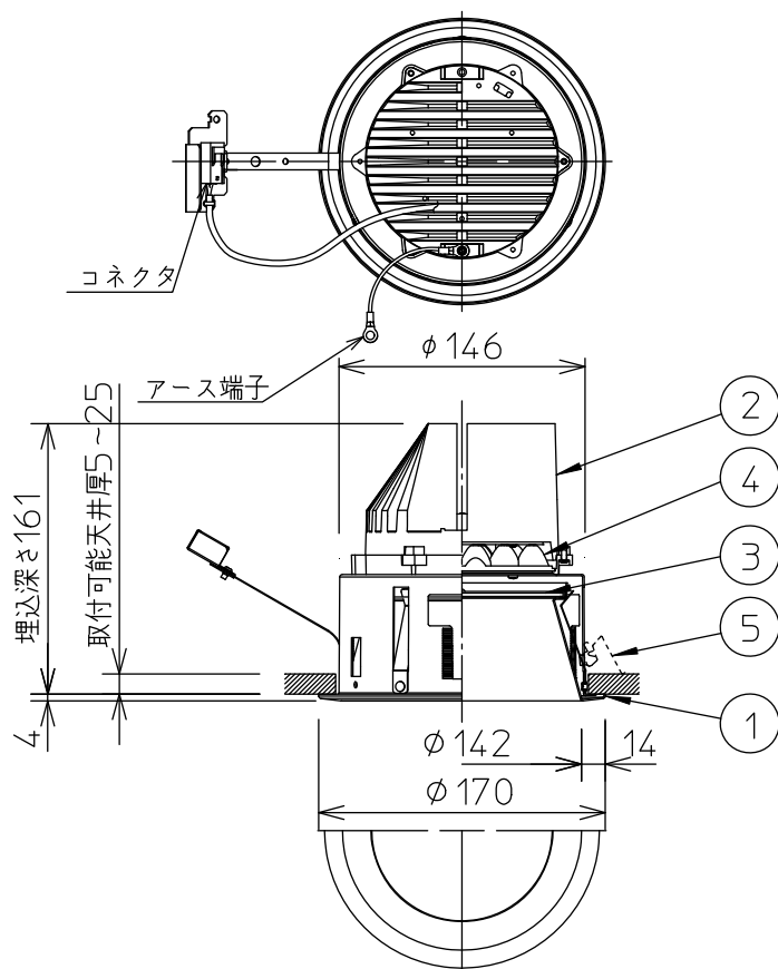
埋込穴寸法
