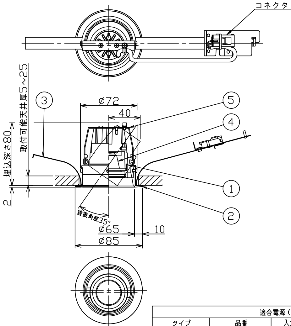
埋込穴寸法
