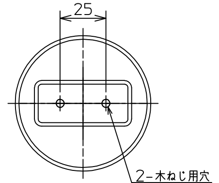
取付部詳細
