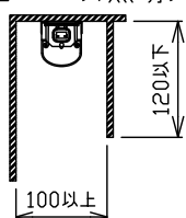
（コーニス照明）
