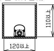
（床面取付密閉）
