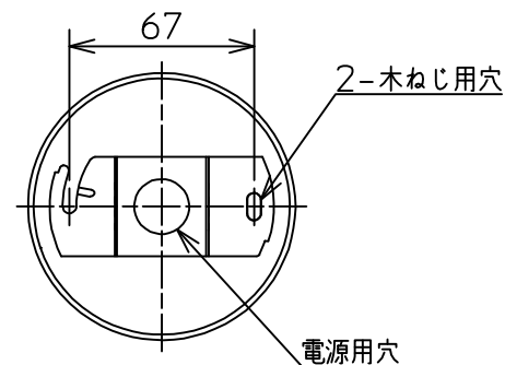
取付部詳細
